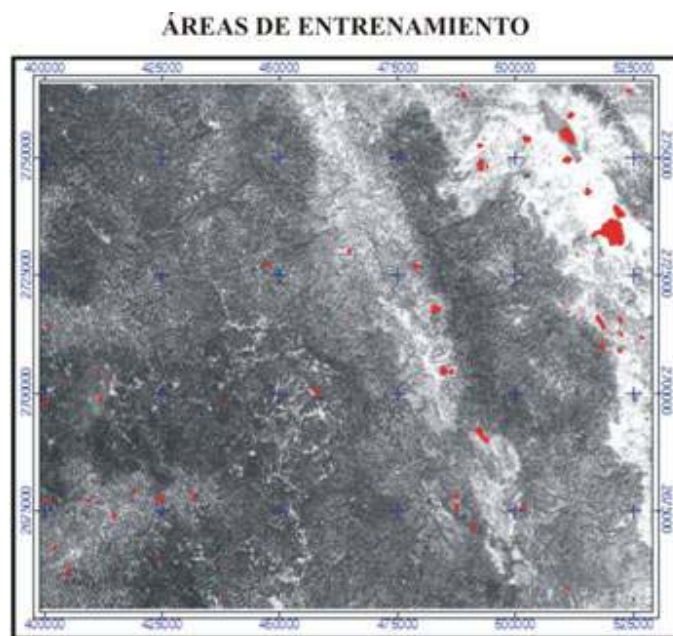
Figura 4. Distribución de las áreas de entrenamiento en color rojo sobre la banda ETM 3.
