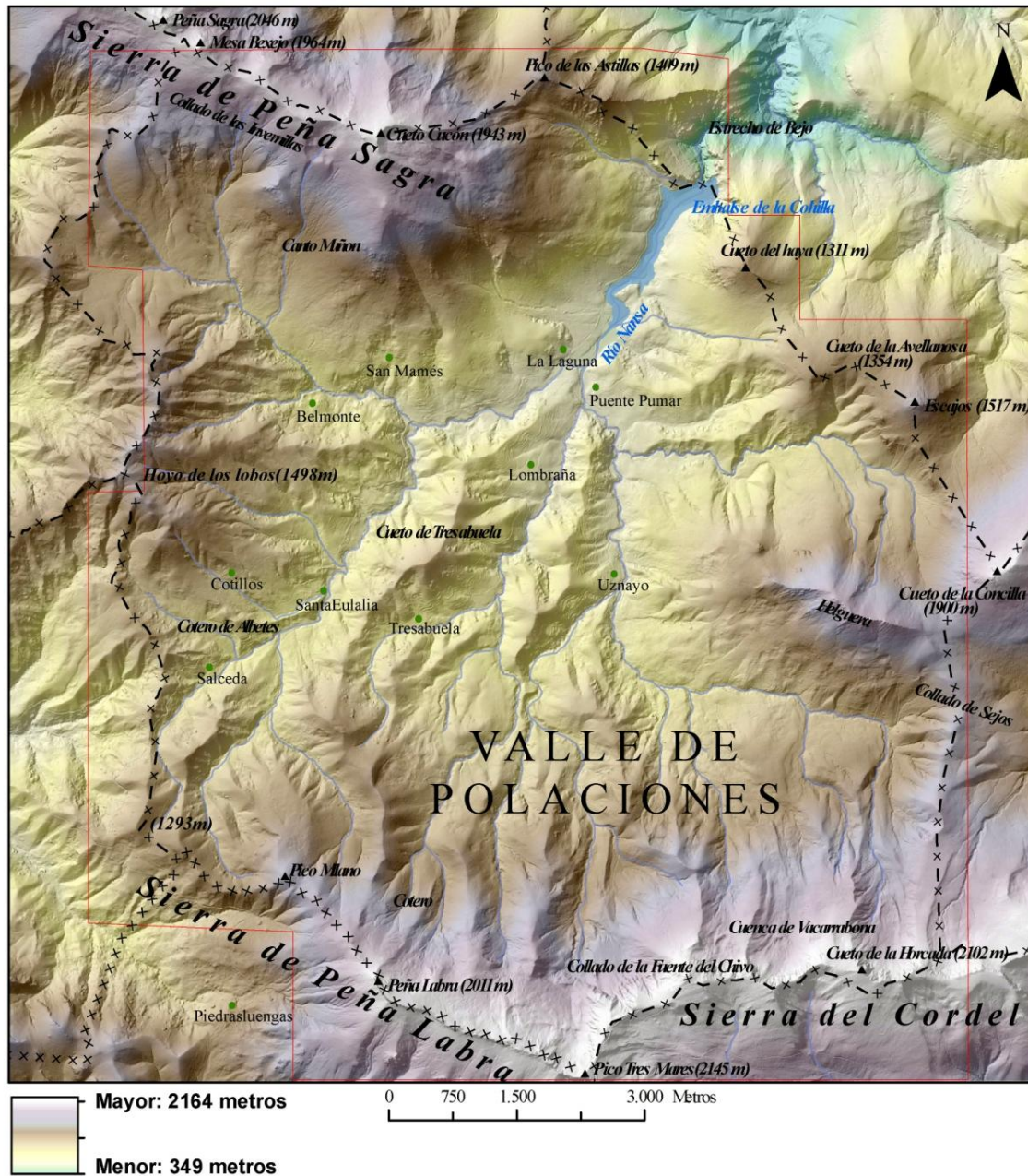
Figura 2. Principales rasgos del área de estudio.
